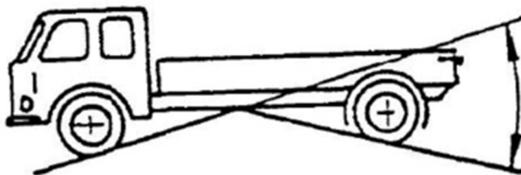
Рисунок 3. Продольный угол проходимости
