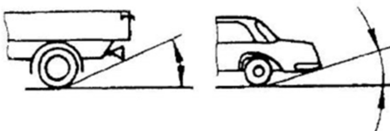
Рисунок 2. Угол съезда
