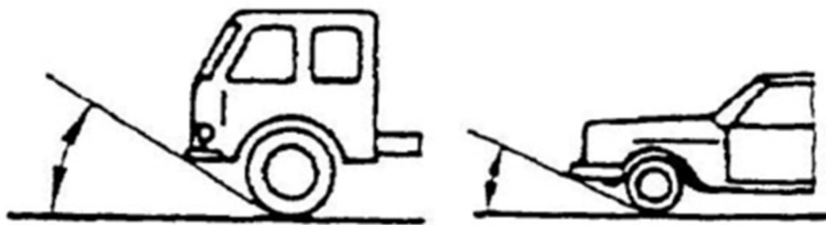
Рисунок 1. Угол въезда
